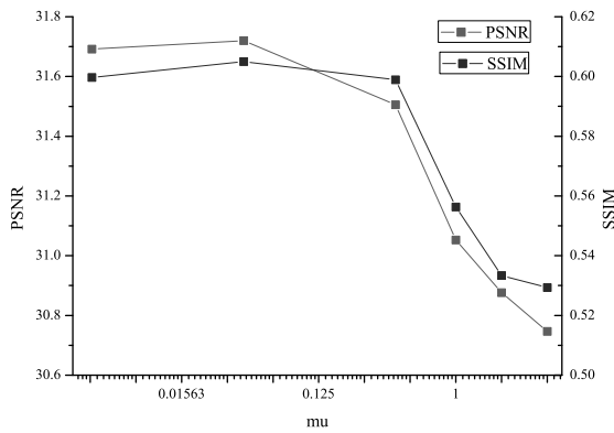
(b) parameter \mu_0
