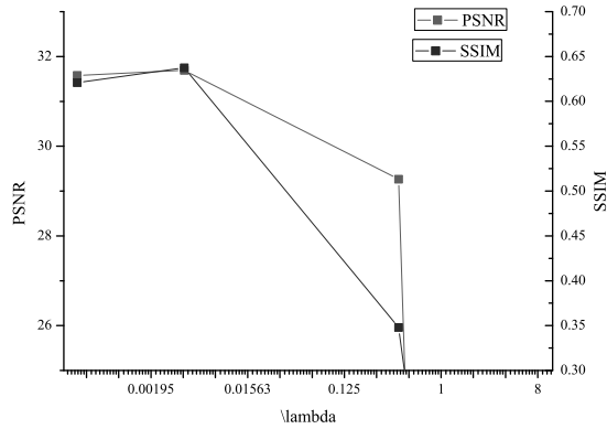
(a) parameter \lambda_0
