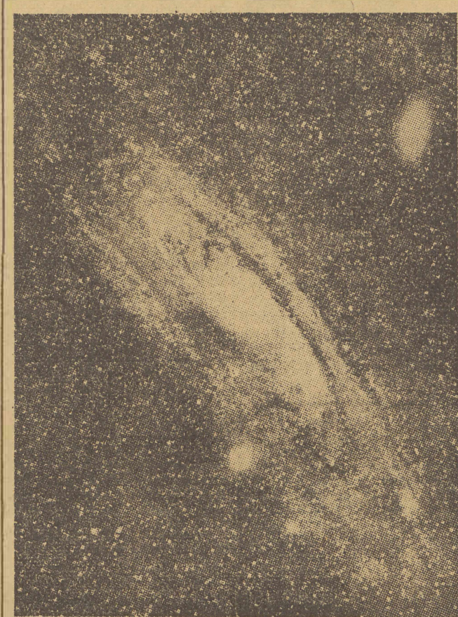
Do największych skupisk materii należy mgławica w Andromedzie. Średnica jej wynosi około 100 tysięcy lat świetlnych. Mgławica ta ma kształt koła od wozu, podobnie, jak i nasza galaktyka. Obrót tej mgławicy dookoła własnej osi wynosi około 20 milionów lat.
