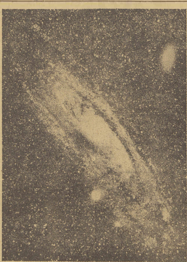
Do największych skupisk materii należy mgławica w Andromedzie. Średnica jej wynosi około 100 tysięcy lat świetlnych. Mgławica ta ma kształt koła od wozu, podobnie, jak i nasza galaktyka. Obrót tej mgławicy dookoła własnej osi wynosi około 20 milionów lat.
