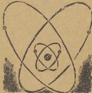
Najdrobniejsza cząsteczka — atom składa się z jądra, posia- dającego dodatni ładunek oraz elektronów, naładowanych u- jemnie wirujących dookoła ja- dra
