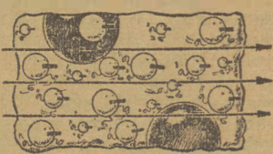
Pod wpływem pola elektrycznego ruch wolnych elektronów w metalach nabiera ciążkości. „Gaz elektronowy” zaczyna działać
