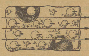
Pod wpływem pola elektrycznego ruch wolnych elektronów w metalach nabiera cięgłości. „Gaz elektronowy” zaczyna działać
