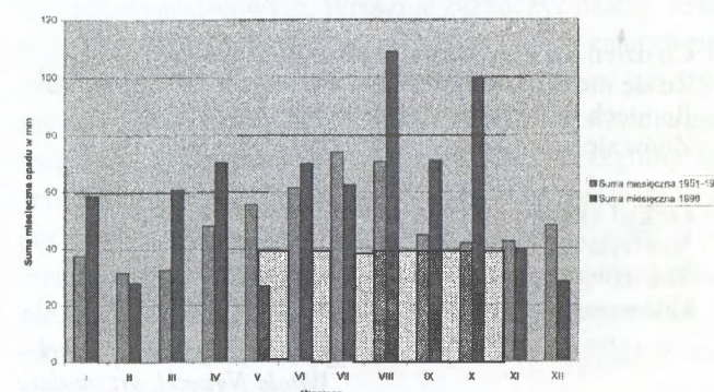
Rys. 2. Średni przebieg roczny opadu na Stacji Meteorologicznej IMGW w Zielonej Górze
