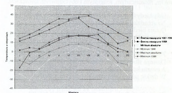
Rys. 1. Przebieg roczny parametrów temperatury powietrza na Stacji Meteorologicznej IMGW w Zielonej Górze
