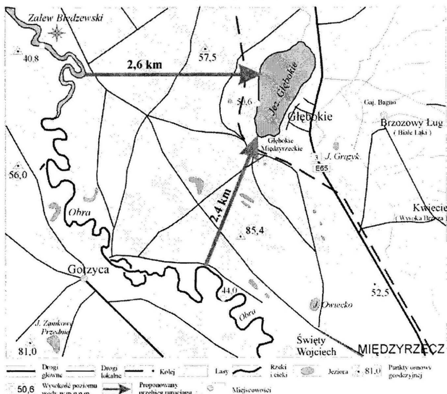
Szkic przebiegu rurociągu do przepompowywania wody z rzeki Obrzy do jeziora Głębokiego - propozycje ( dwa warianty )
