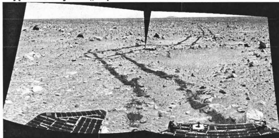
Powyżej „rzut oka” na ledwo widoczny lądowisk odległy o 240m. Zdjęcia do tej mozaiki wykonał 6 marca SPIRIT
