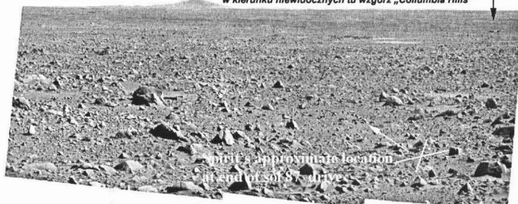
Poniższą panoramę wykonano zaraz przed opuszczeniem krawędzi krateru Bonneville przez SPIRIT'a i wyruszeniem w kierunku niewidocznych tu wzgórz „Columbia Hills”
