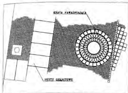
SZCZEGÓŁ A - ZABEZPIECZENIE PNI DRZEW ZA POMOCĄ KRAT NAWADNIAJĄCYCH
