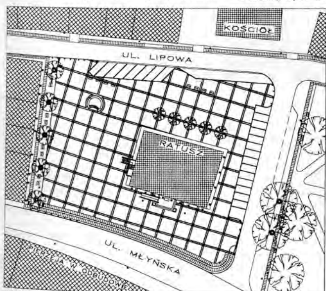
RZUT RYNKU ZE SCHEMATEM UKŁADU NAWIERZCHNI
