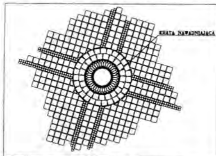
SZCZEGÓŁ C - ZABEZPIECZENIE PNI DRZEW ZA POMOCĄ KRAT NAWADNIAJĄCYCH
